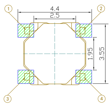
P.C.B. Land Patten
